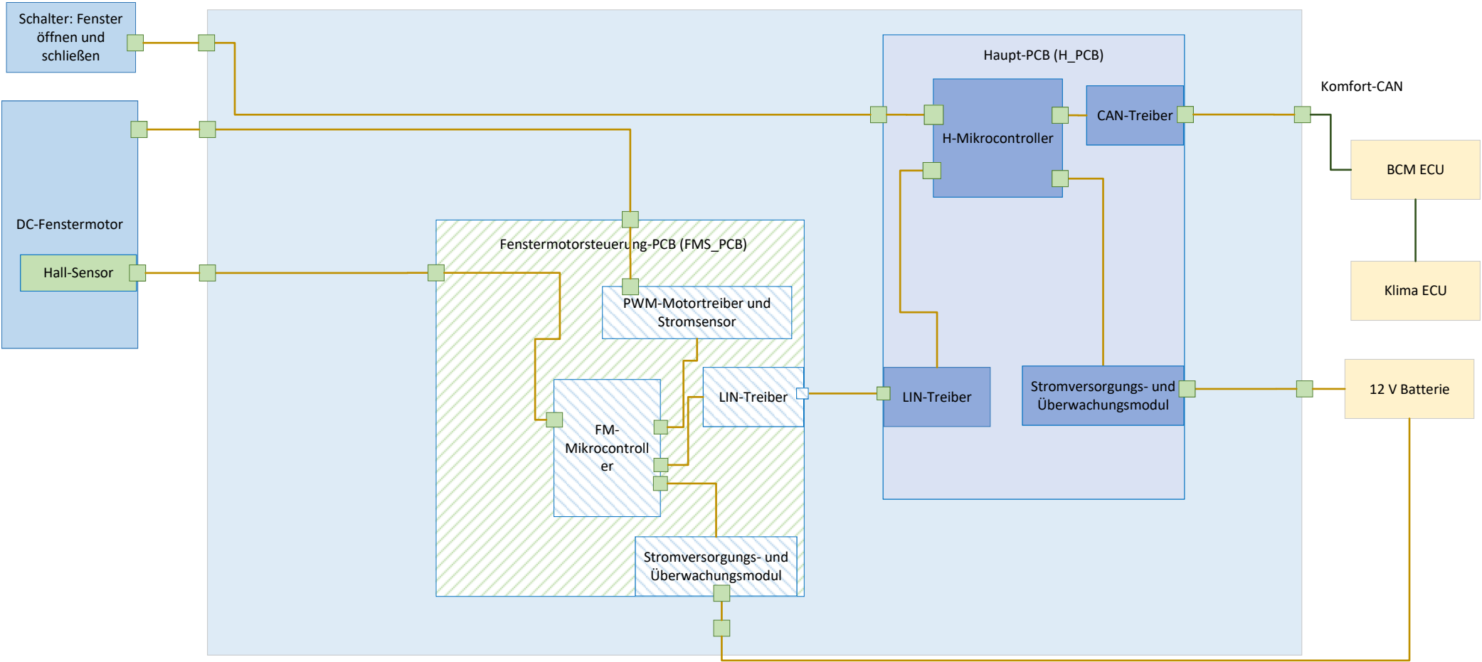
Fensterheber ECU – FMS_PCB-Kontext (High-Level-Systemarchitektur)
